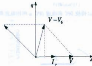
(a) 传统 ST-DPC 矢量合成图
